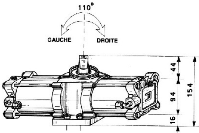
VERIN
