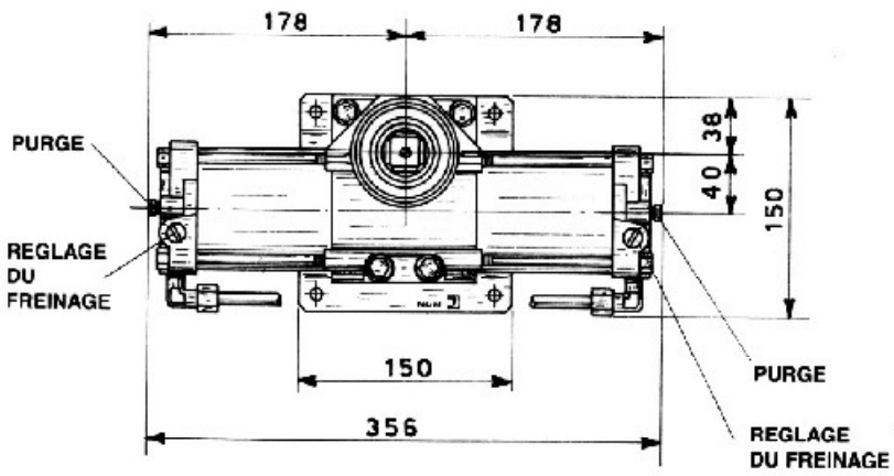
VERIN
